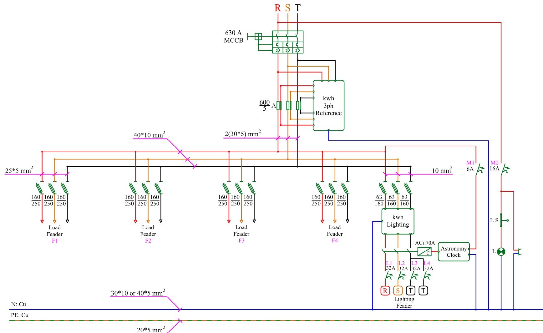
شکل ۹: دیاگرام تک خطی تابلوهای توزیع عمومی بارانی ۶۳۰ آمپری
