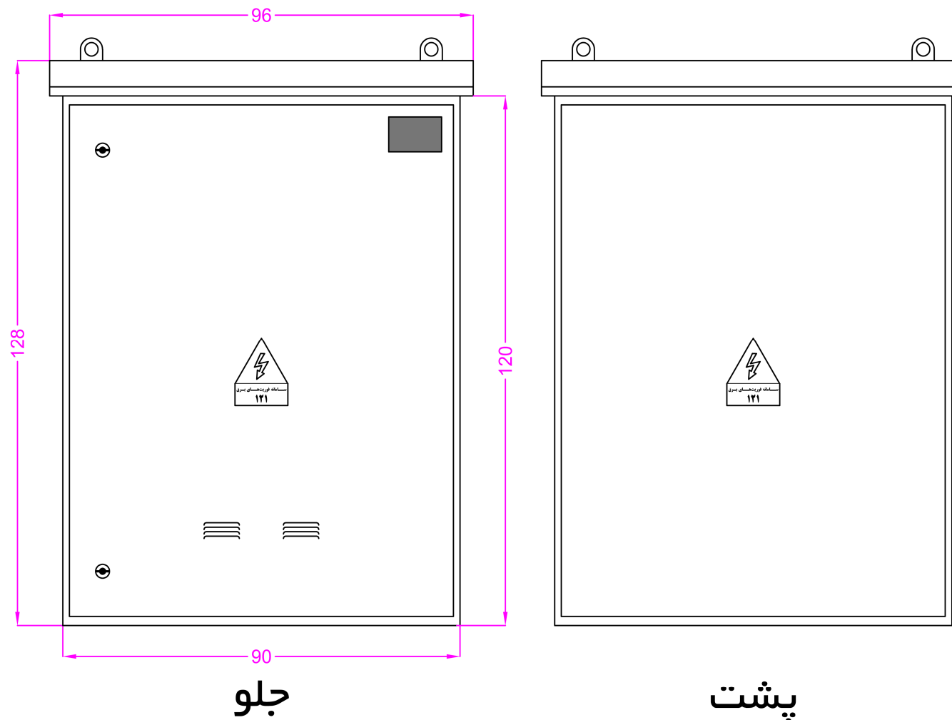
شکل ۳: نمای خارجی تابلوهای توزیع عمومی بارانی ۶۳۰ آمپری - جلو و پشت
